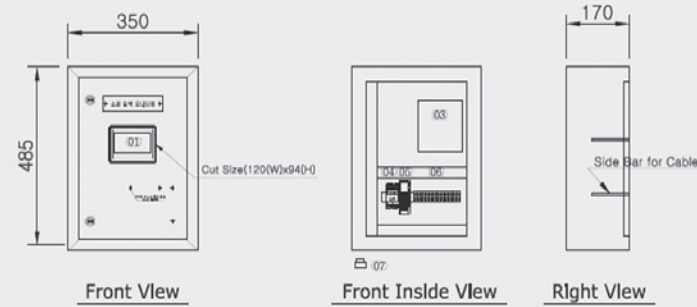
(2) (모델명: VPM-SP-02)
